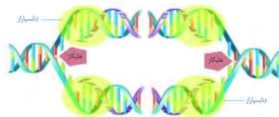
شکل ۱۱- همانندسازی دنا
