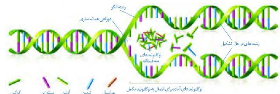
شکل ۱۲- همانندسازی دنا
