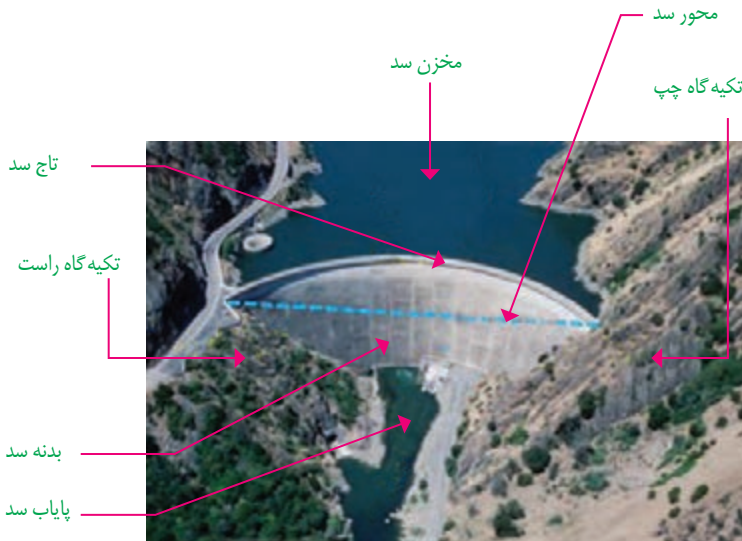
شکل ۱۸-۶- نمایه بخش‌های مختلف یک سد را نام ببرید 57
